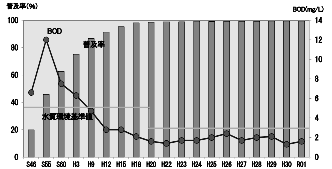
図表4-5 下水道普及率と多摩川の水質の推移
