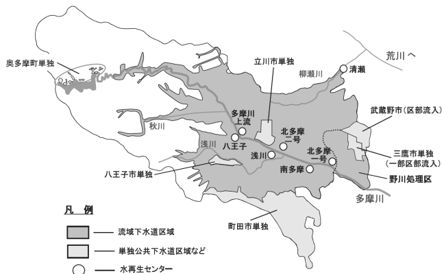
図表4-2 多摩地域の下水道計画区域の構成
