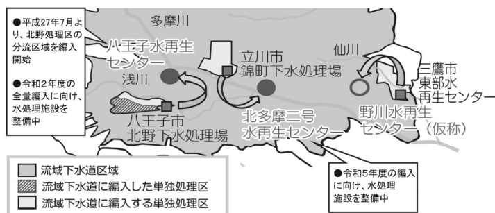
図表4-27 単独処理区の編入計画
