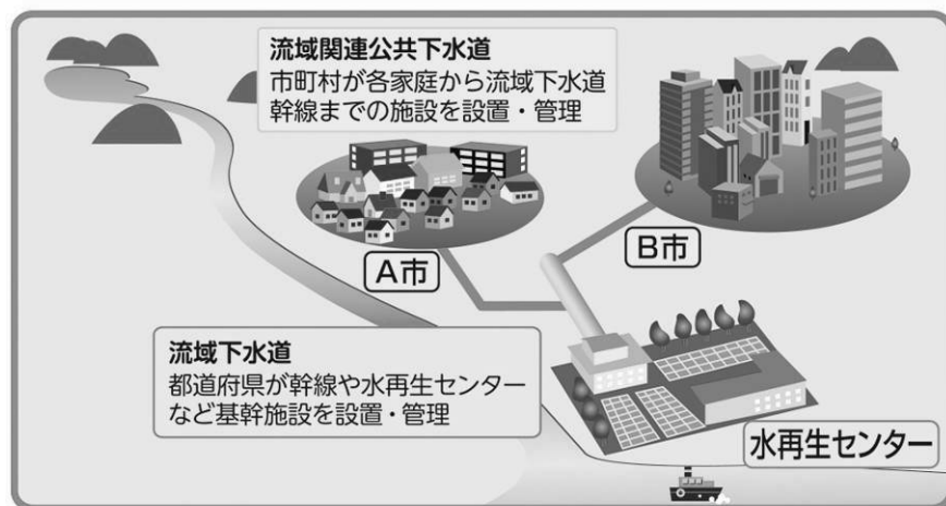
図表4-1 流域下水道のしくみ
