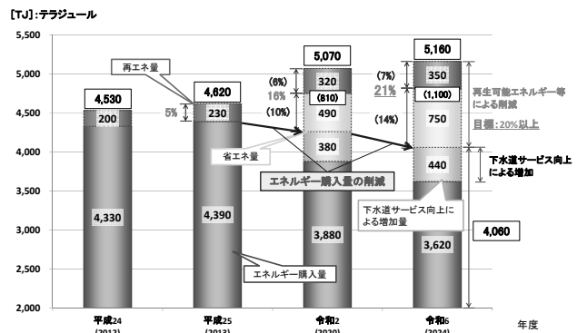
図表5-8 新たな取組による今後の総エネルギー使用量の見込み
