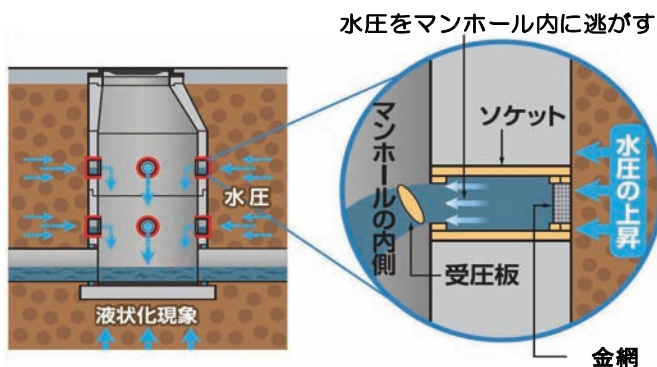
マンホールの浮上抑制対策
