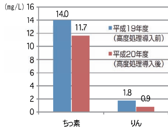
図表3-3 砂町水再生センターにおける高度処理導入に伴うちっ素、りん濃度の状況
