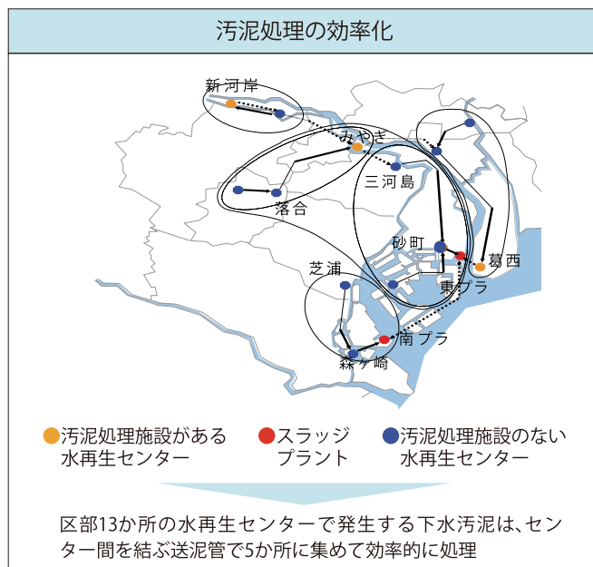
図表3-2 汚泥処理の集約化
