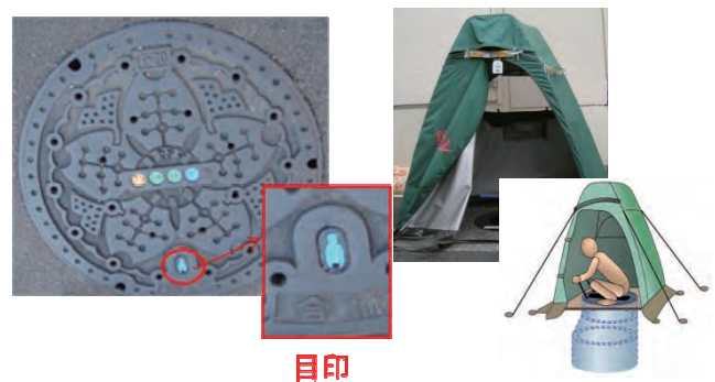
図表6-2 仮設トイレの設置が可能なマンホール及び仮設トイレ
