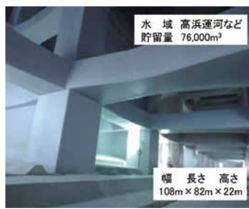
貯留施設（芝浦水再生センター）
